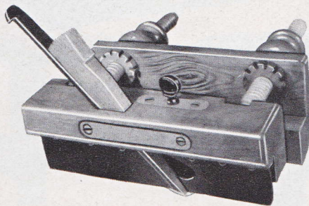
N° 53 BOUVET 2 PIÈCES A APPROFONDIR DESCENTE A POMPE, TIGE A VIS
